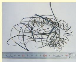
ブレイクマスターSV型 BNC200 (ブレーカなし) 他社CBN (ブレーカ付き)
