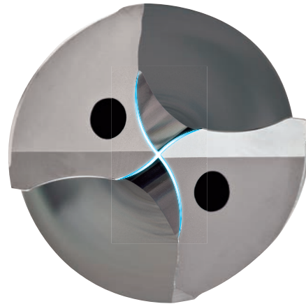
内部給油式
