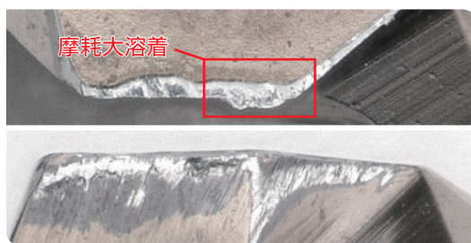
900穴加工後
