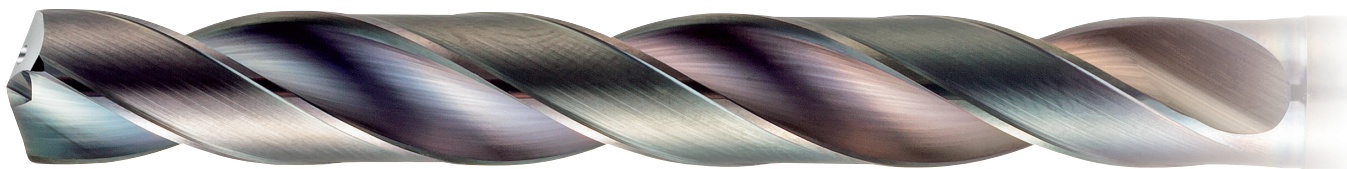
内部給油式：ダブルマージン
