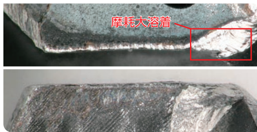
3,840穴加工後
