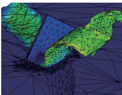
切りくずシミュレーション
